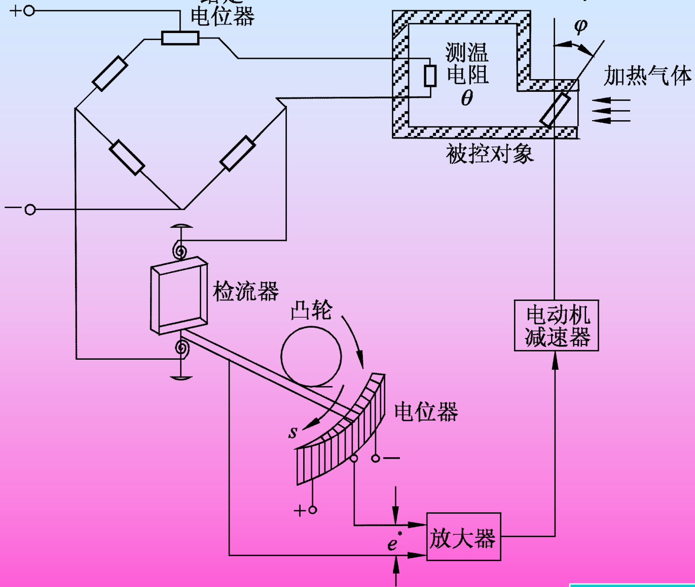
炉温采样控制系统原理图
