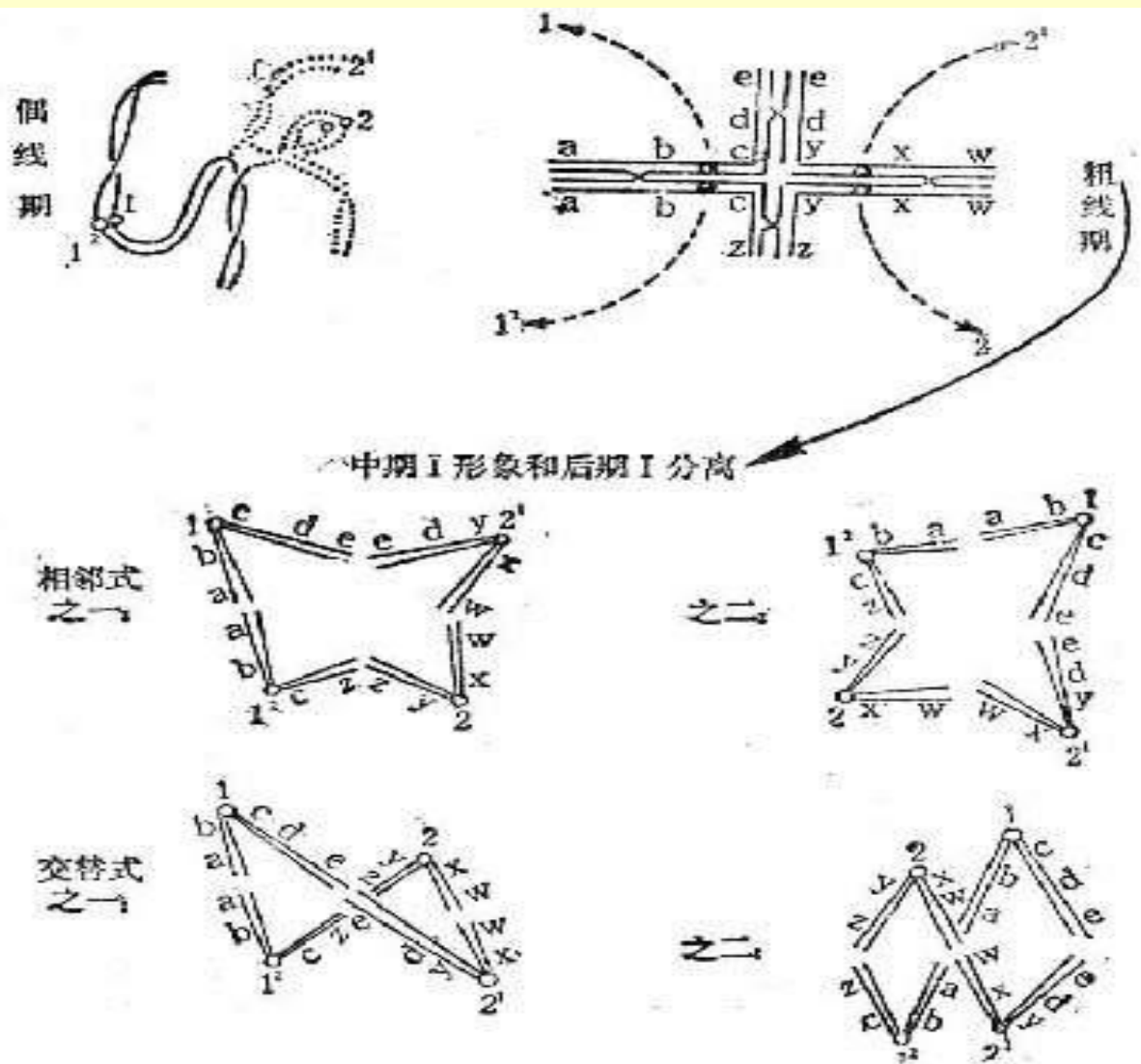
图 8—9 易位杂合体的联会和分离示意图
